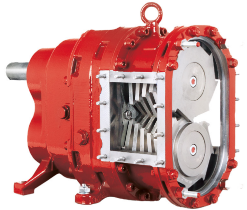
Vogelsang XRipper
