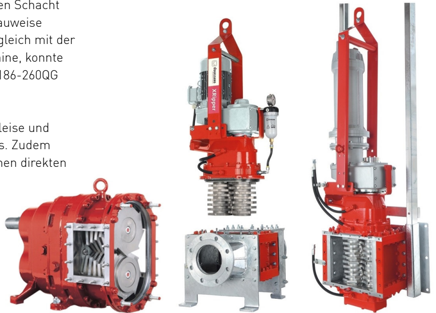
Der Abwasser-Zerkleinerer XRipper von Vogelsang
