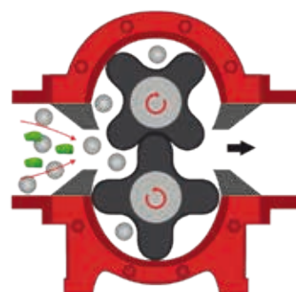
Lobbenpomp met InjectionSystem
