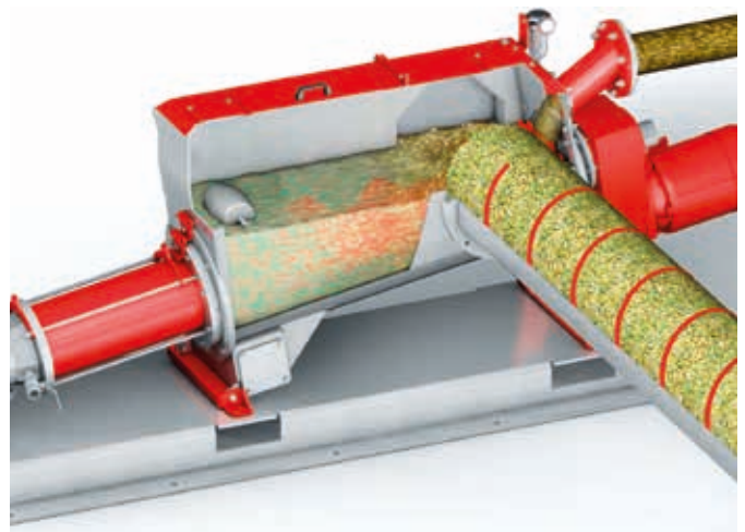
Section d'un CC-Mix, à droite sur l'image : alimentation en matière solide via une vis d'alimentation
