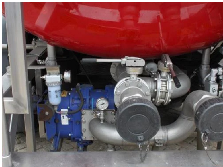
Cisternový vůz s čerpadlem s rotačními písty řady VX od společnosti Vogelsang
