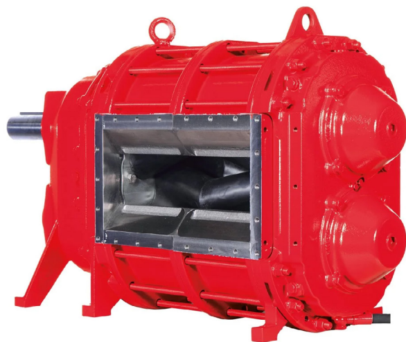
Čerpadlo s rotačními písky od společnosti Vogelsang
