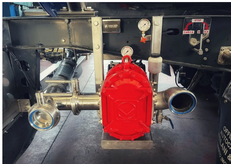
Čerpadlo s rotačními písky - VX136-140Q se systémem ASU
