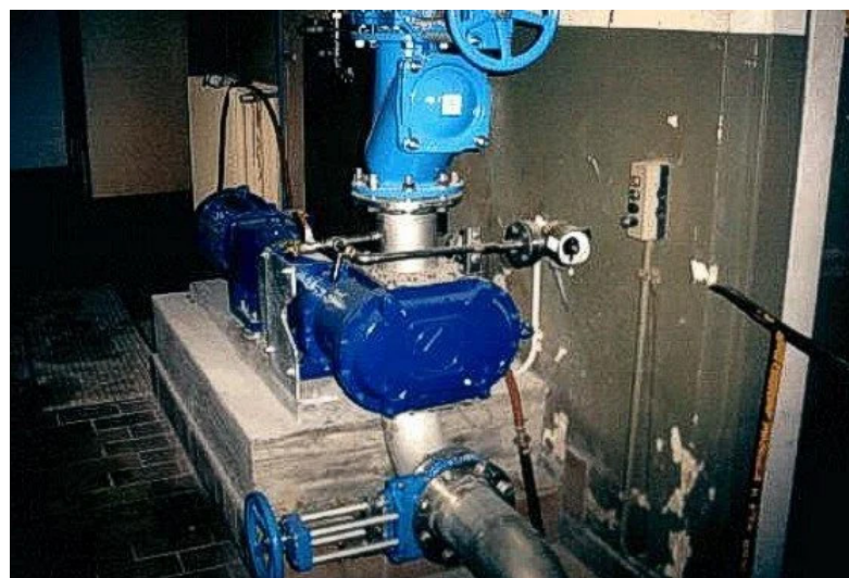
Lobbenpomp VX186-260Q van Vogelsang
