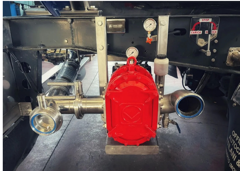
Bomba lobular rotativa - VX136-140Q con sistema ASU
