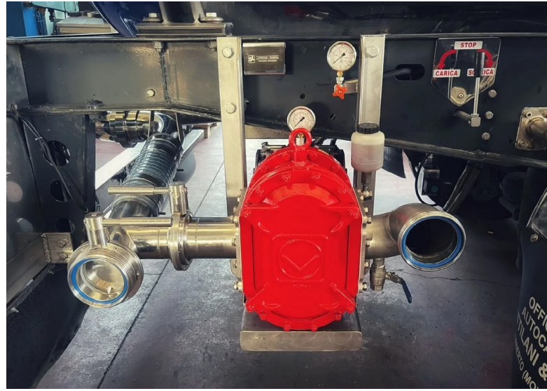
带 ASU 系统的 VX136-140Q 转子泵
