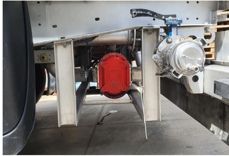
福格申VX136-210Q转子泵 (双液压马达驱动型)
