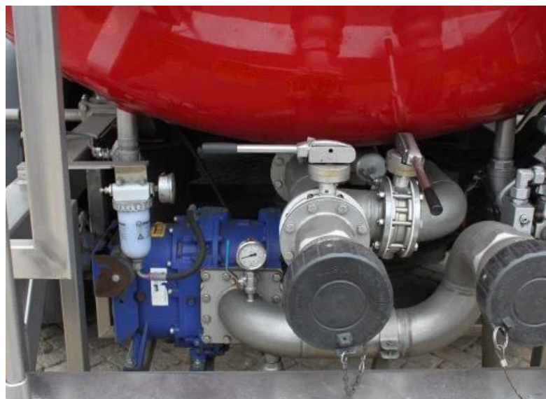
配备福格申VX系列转子泵的罐式卡车
