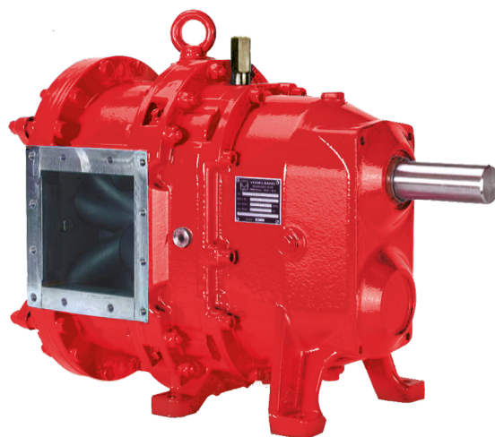
Vogelsang VX136
