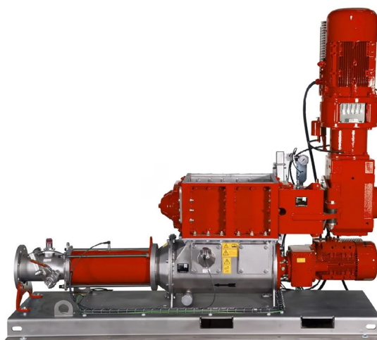
RedUnit system med dobbelakslet RedUnit XRL neddelers og CC serie progressiv skruepumpe til effektiv neddeling og pumpning af fjerkræaffald
