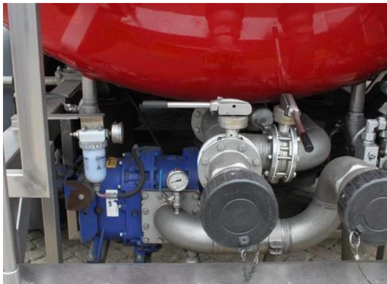
Tankbil med Vogelsang rotationspumpe i VX serien
