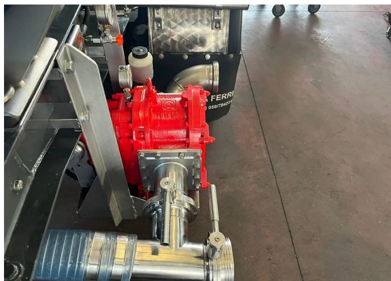
Vogelsang rotationspumpe i fødevarerapplikation
