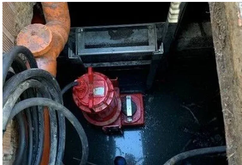
Neddykket installation, der finder plast og klude før pumpen og sikrer stabil drift uden lugtgener
