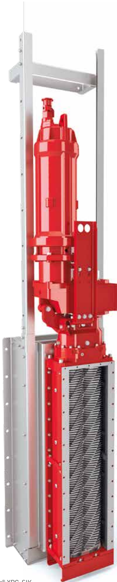
XRipper® XRC-SIK
